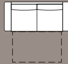
SOF.3S 160 VISCO 228 / 102 / 91 Sofa z funkcją spania z materacem VISCO, nie posiada pojemnika, pow. spania 160 x 196 Sofa with sleeping function with VISCO mattress, does not have a bedding container, sleeping area 160 x 196
