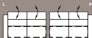
SEGM.2P N/CR L/P 158/98/87-101 SEGM.2P CR1 L/P SEGM.2P CR2 L/P Element modułowy, wybierz stronę lewą lub prawą Modular element, choose the left or right side
