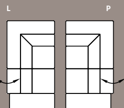
SEGM.20T N/CR L/P 100/180/87-101 SEGM.20T CR1 L/P SEGM.20T CR2 L/P Element modułowy bez pojemnika, wybierz stronę lewą lub prawą Modular element without bedding container, choose the left or right side
