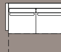
SOF.3R 217/110/95 Sofa z funkcją spania, z pojemnikiem, pow. spania 154 x 200cm, w cenie 4 poduszki oparciowe Sofa with sleeping function, with bedding container, sleeping area 154 x 200 cm, price includes 4 backrest pillows
