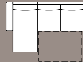
NAR.3S/10T 140 HR 293x175/102/91 Moduł z funkcją spania z materacem HR, z pojemnikiem, pow. spania 140 x 196, wybierz stronę narożnika Module with sleeping function with HR mattress, with container, sleeping area 140 x 196, choice of corner side
